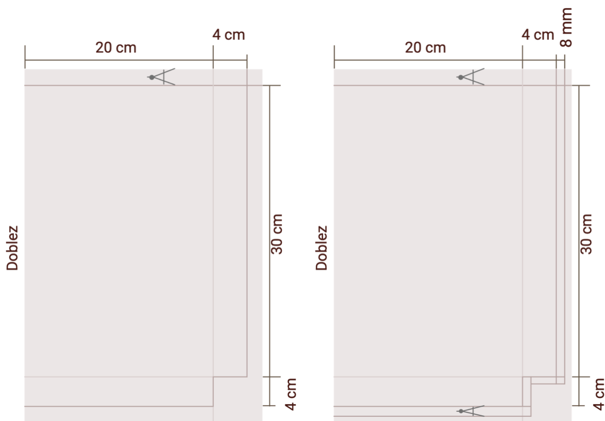
Figura 12. Trazado de pinza
