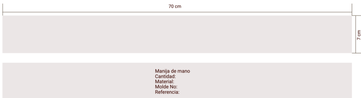
Figura 27. Molde manija plana
