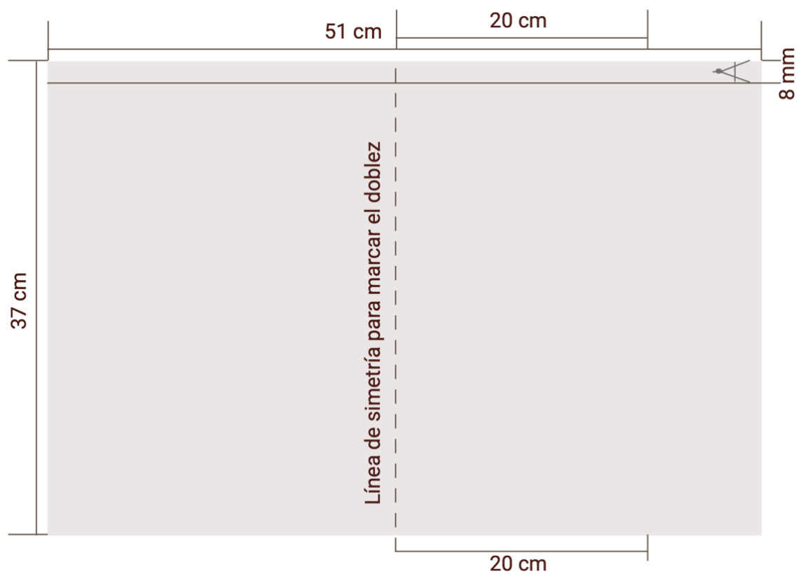
Figura 10. Molde para agregar ventaja de costura
