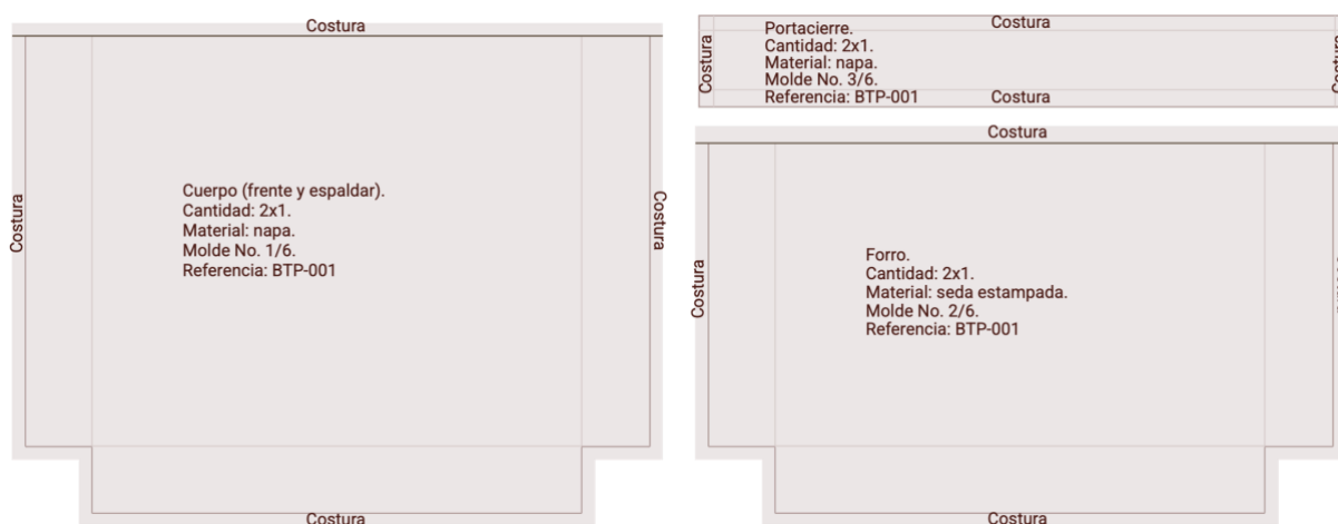
Figura 26. Industrialización de los moldes
