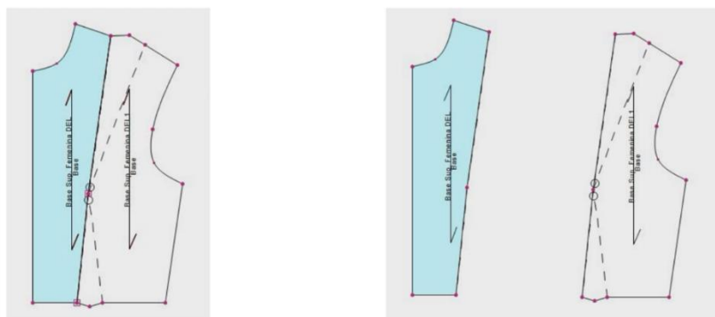
Figura 79. Identificación de las piezas resultantes y de los hilos de tela independientes después del corte.
