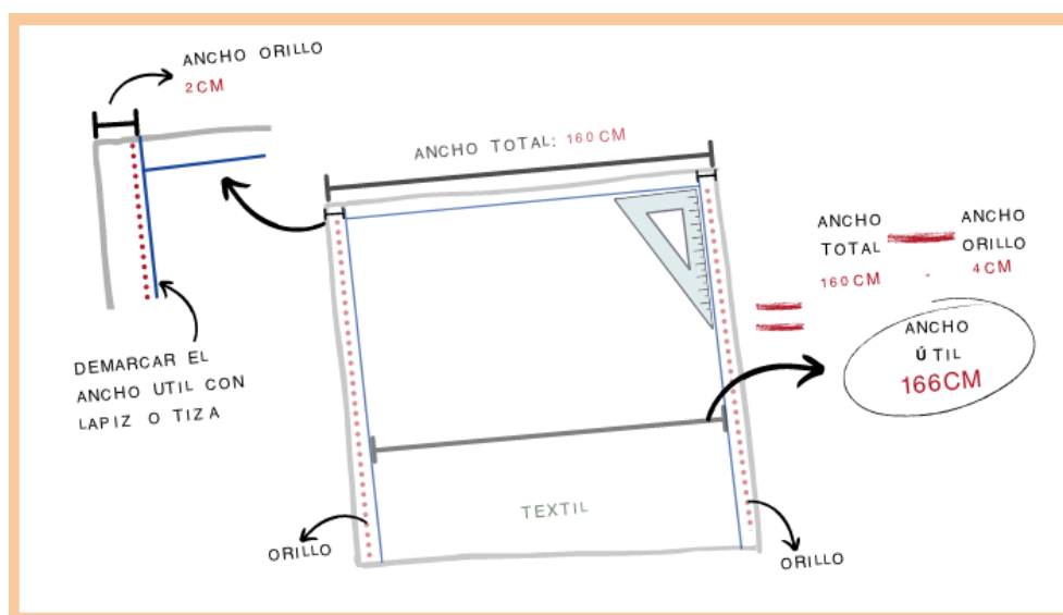
Figura 165. Cálculo del ancho útil de la tela a partir del ancho total y los orillos
