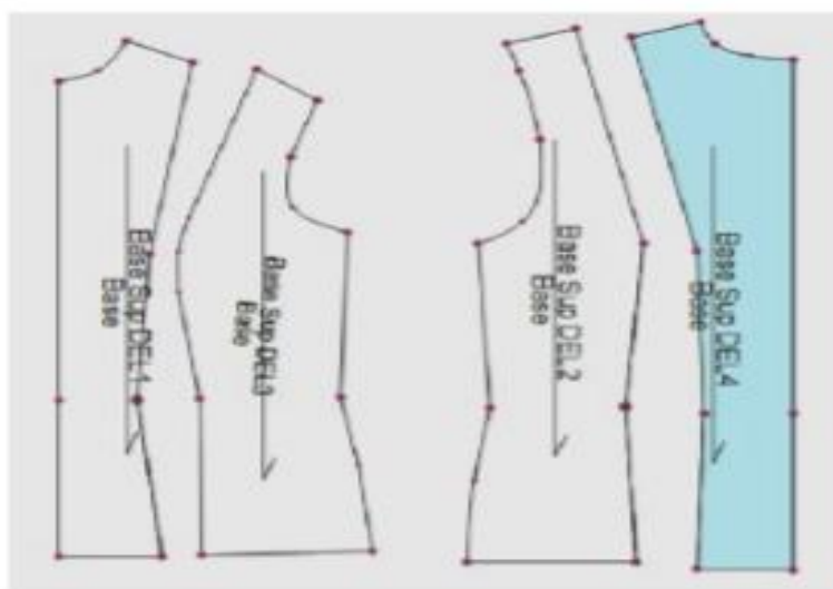
Figura 126. Generación del corte princesa en la espalda
