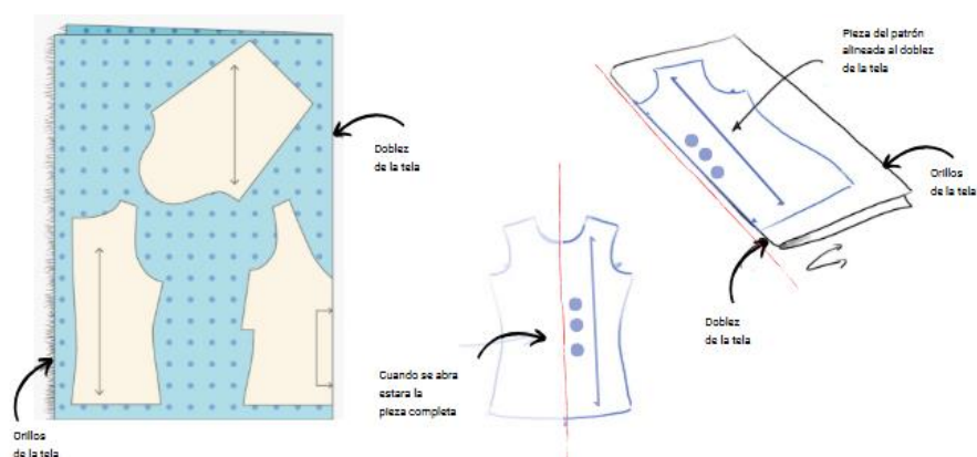
Figura 155. Distribución de piezas en tendido cerrado alineadas al dobléz y al orillo de la tela
