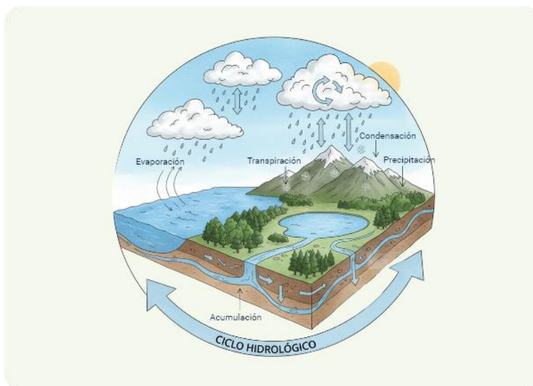
Figura 1. Ciclo hidrológico
