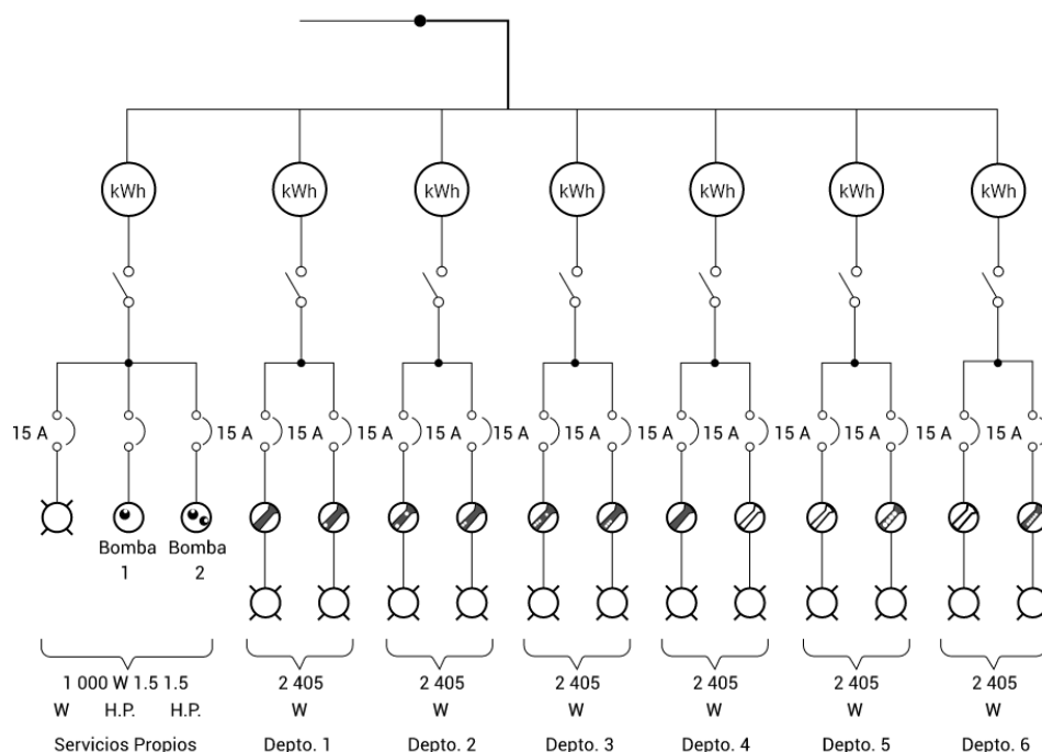
Figura 4. Plano de diagrama unifilar
