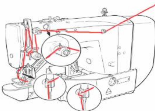
Figura 31. Enhebrado de la máquina
