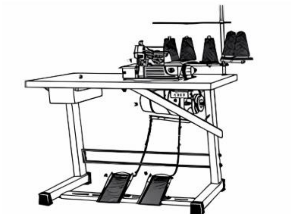
Figura 20. Pedales máquina fileteadora
