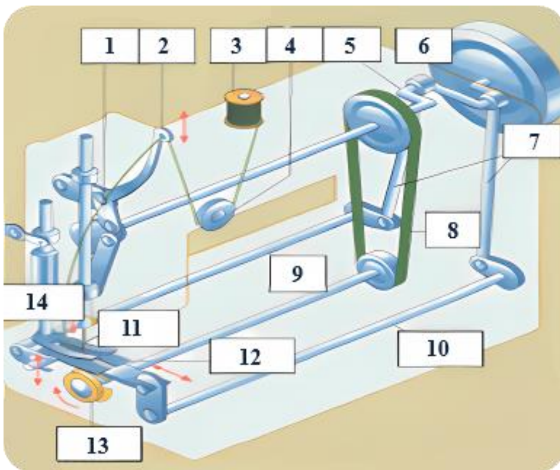
Figura 5. Máquina de coser
