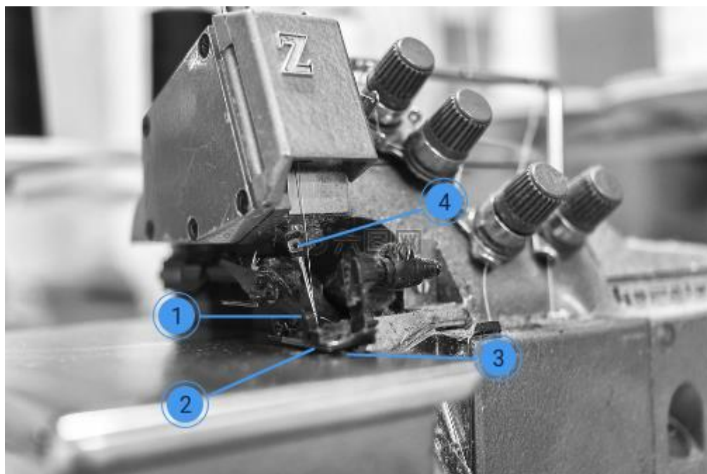
Figura 44. Ajuste fileteadora
