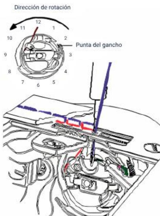
Figura 17. Mecanismo de formación de la puntada
