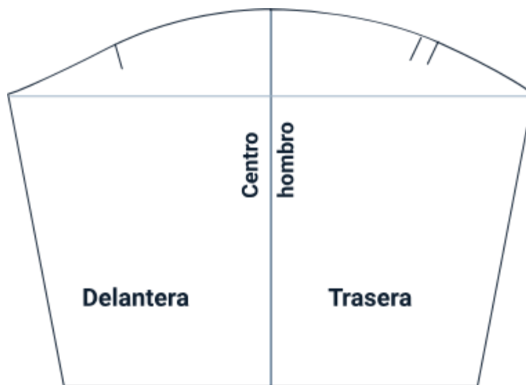
Figura 33. Despiece de la manga de la camiseta
