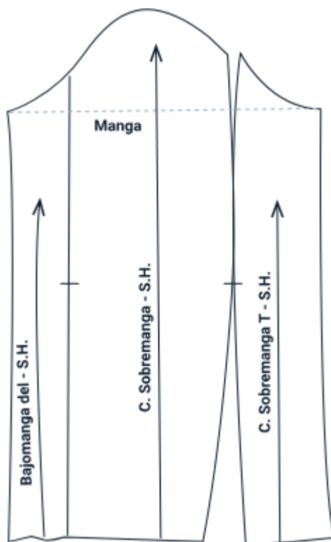
Figura 26. Trazo del patrón de la manga de la chaqueta
