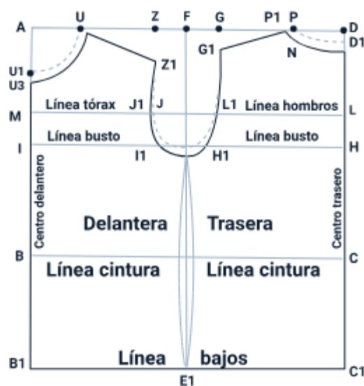
Figura 30. Trazo de la camiseta
