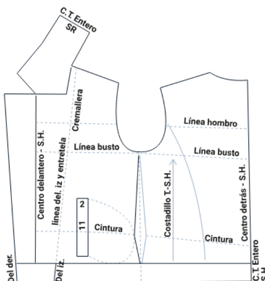
Figura 25. Trazo del patrón delantero y posterior de la chaqueta
