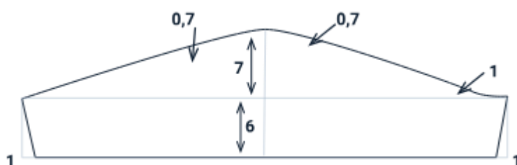
Figura 6. Trazo del patrón de la manga
