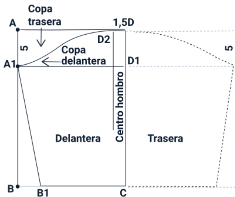
Figura 31. Trazo del patrón de la manga
