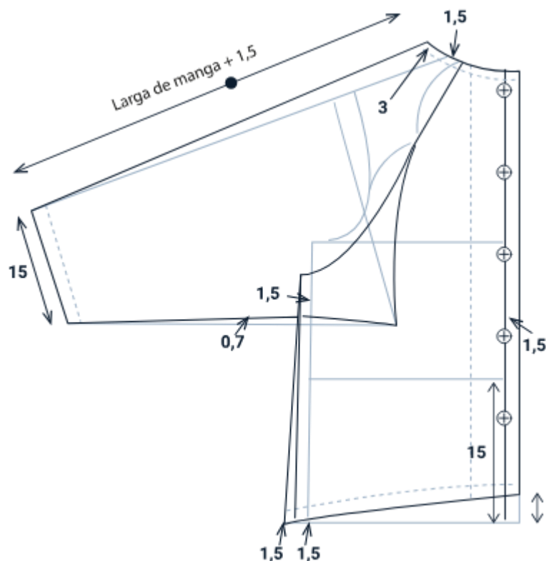
Figura 19. Trazo del patrón del posterior de la blusa manga raglán
