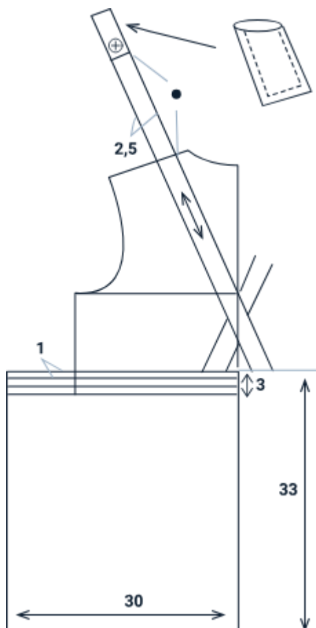
Figura 23. Trazo del patrón del posterior de la jardinera
