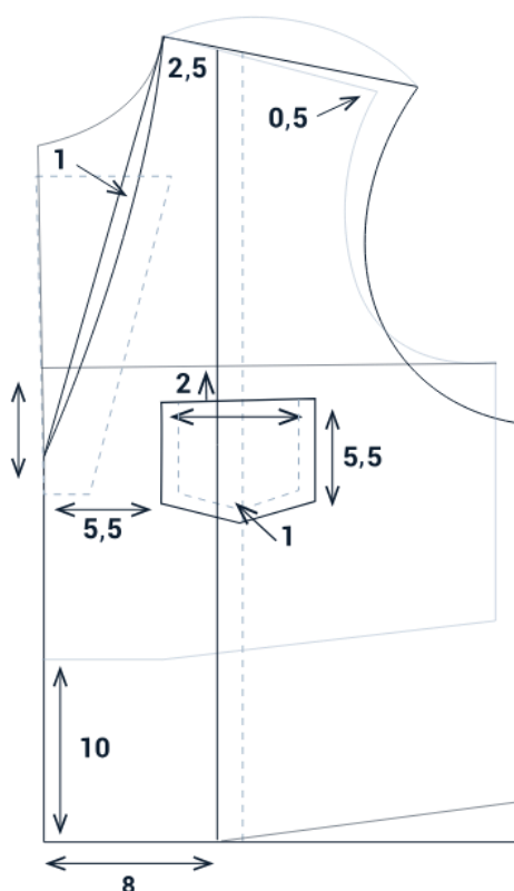
Figura 2. Trazo del delantero
