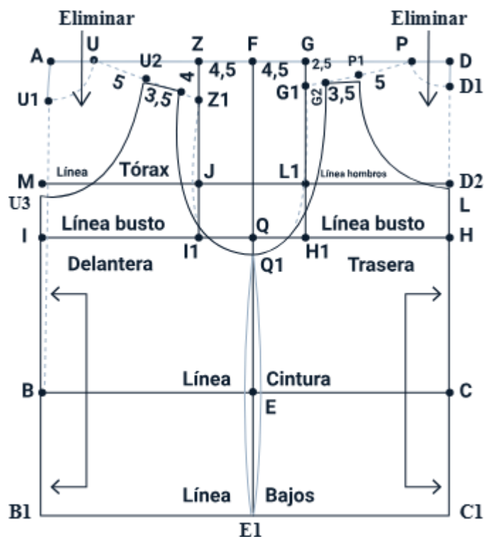
Figura 28. Trazo de la camisilla
