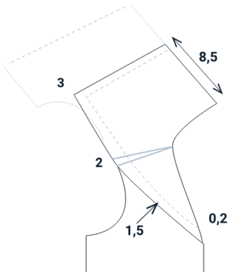
Figura 5. Trazo del patrón del cuello marinero
