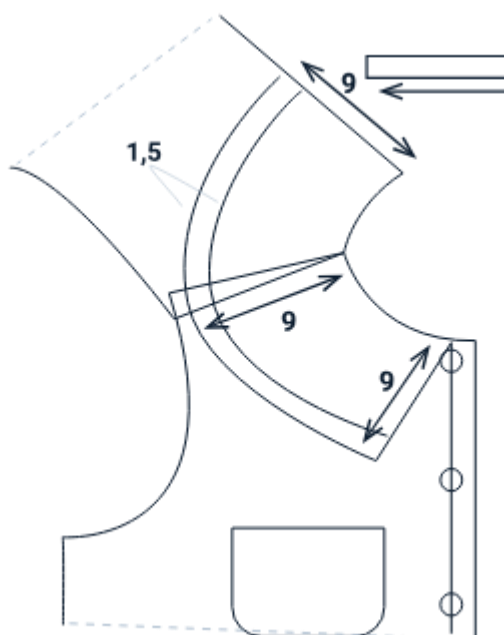
Figura 12. Trazo del molde del cuello bebé
