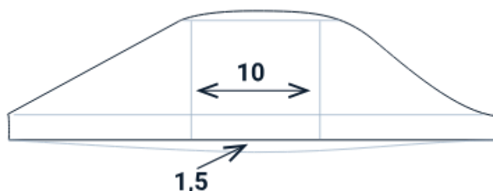
Figura 10. Trazo del patrón de la manga
