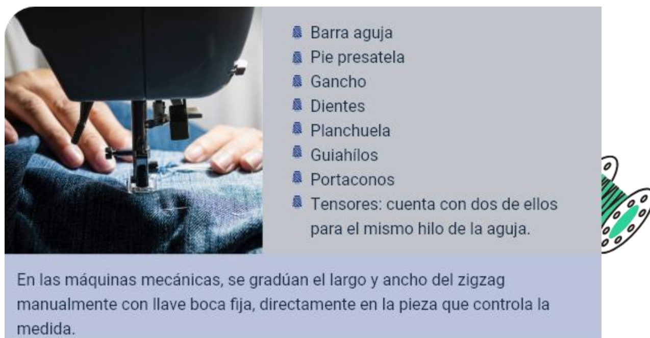
Figura 4. Partes presilladora.
