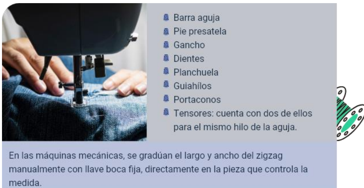
Figura 4. Partes presilladora.
