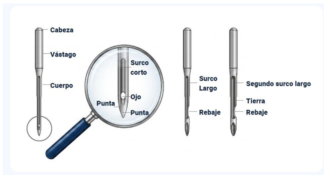
Figura 6. Partes de la aguja.
