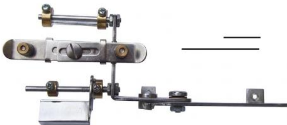
Figura 10. Dosificador de elástico y tipo de costura.
