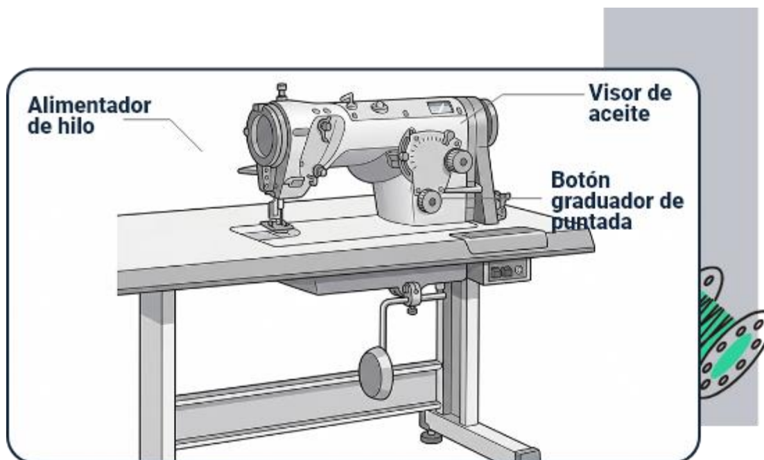
Figura 3. Partes de la máquina zigzadora Brother ZM-851A.
