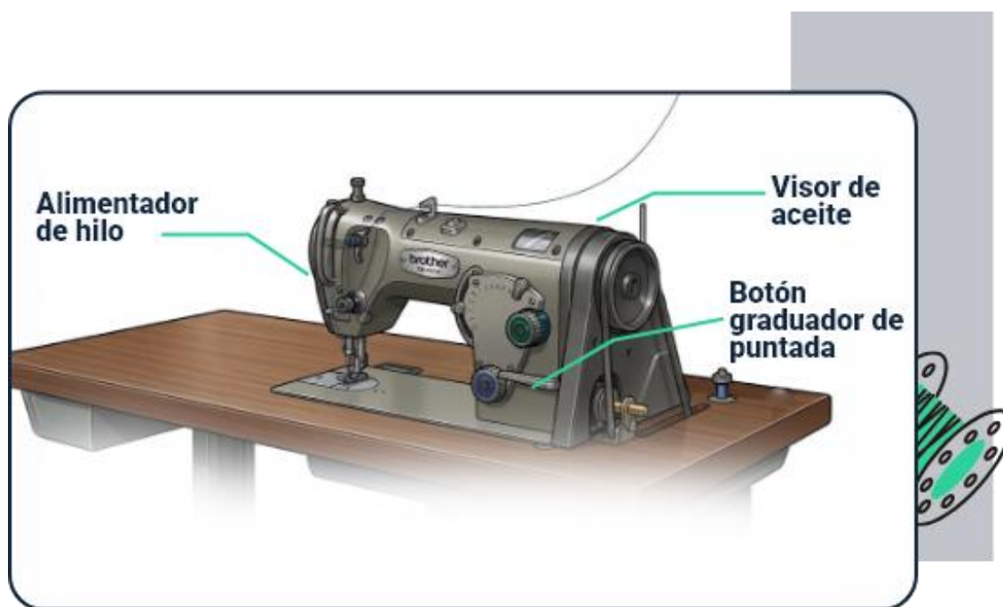
Figura 4. Partes de la máquina zigzadora Brother ZM-851A.
