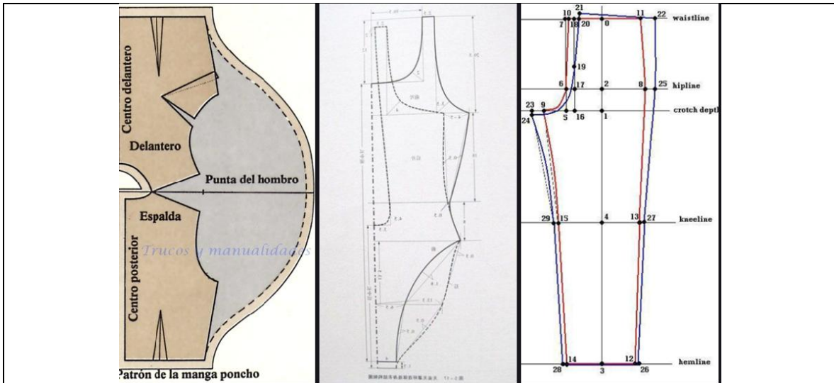
Figura 11. Planos de unión
