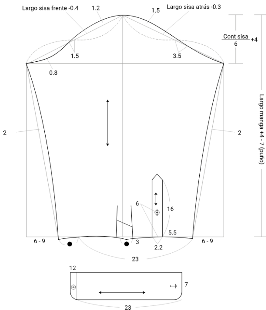
Figura 11. Trazo del plano de la manga slim fit
