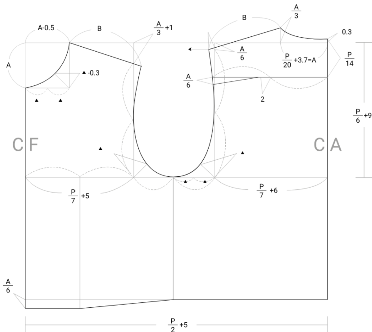
Figura 7. Base masculino slim fit
