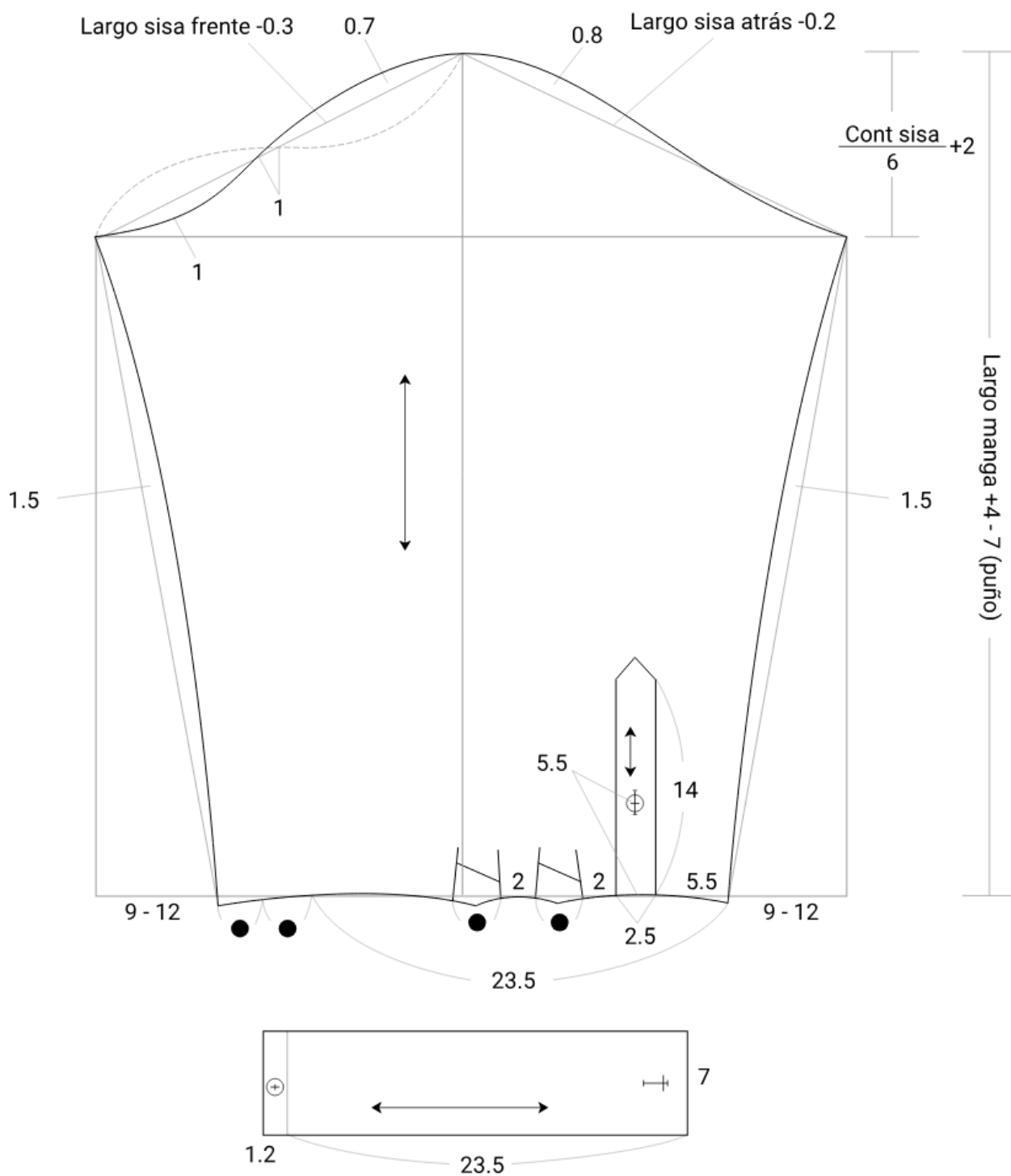
Figura 9. Trazo base manga clásica
