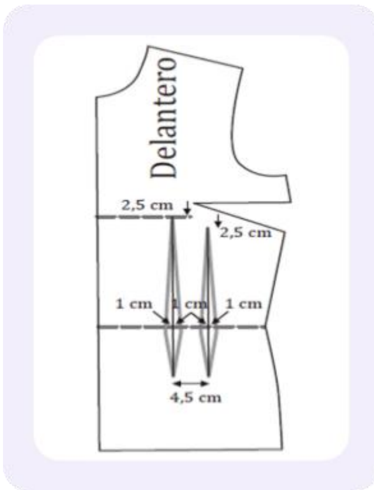
Figura 31. Quinto paso para el trazo
