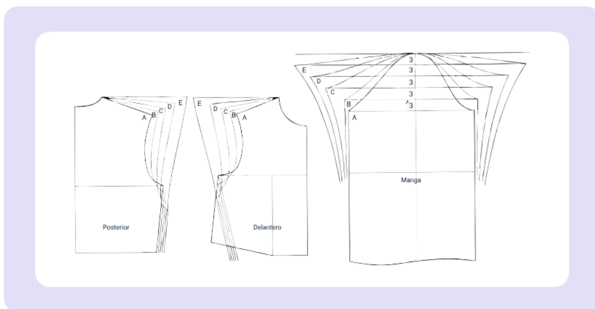
Figura 22. Transformaciones de sisas según tipo de manga
