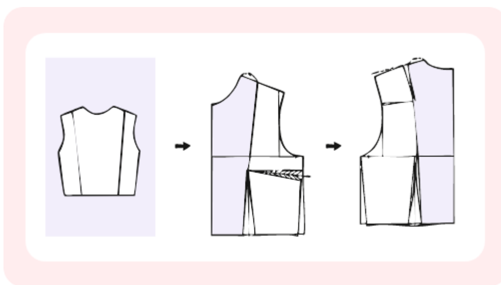
Figura 38. Crop top con corte princesa
