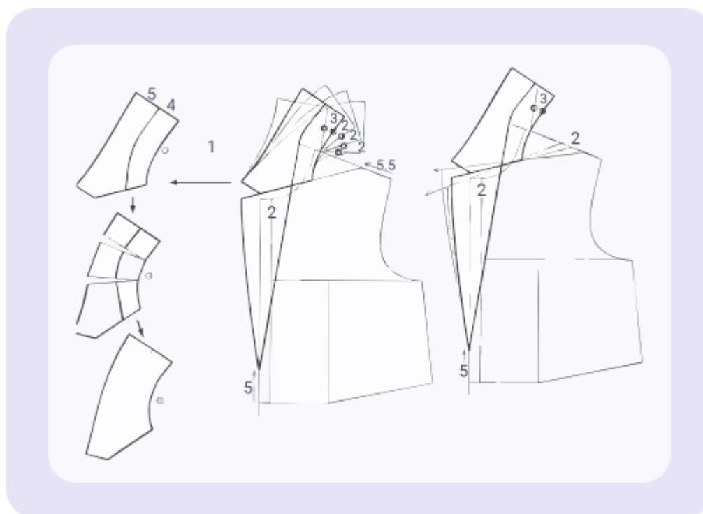
Figura 19. Cuello y solapa
