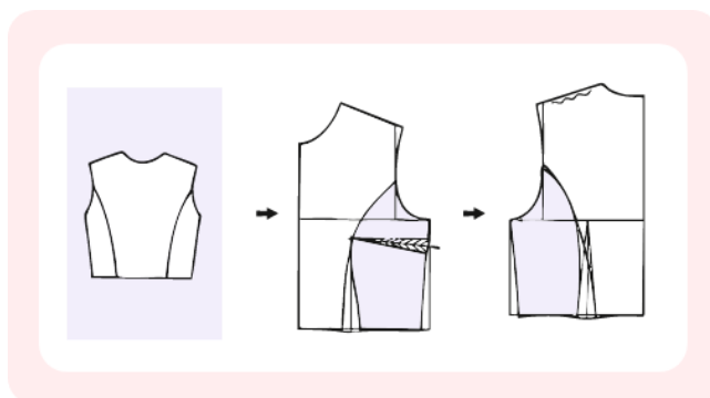
Figura 39. Crop top con corte princesa en sisa
