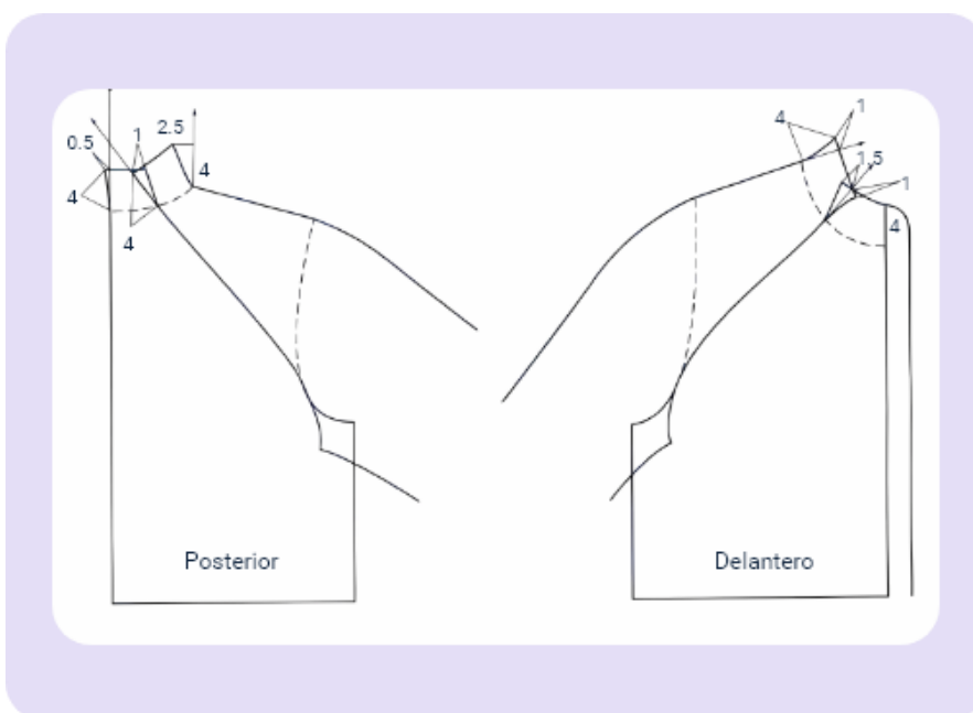
Figura 20. Cuello alto con manga raglán
