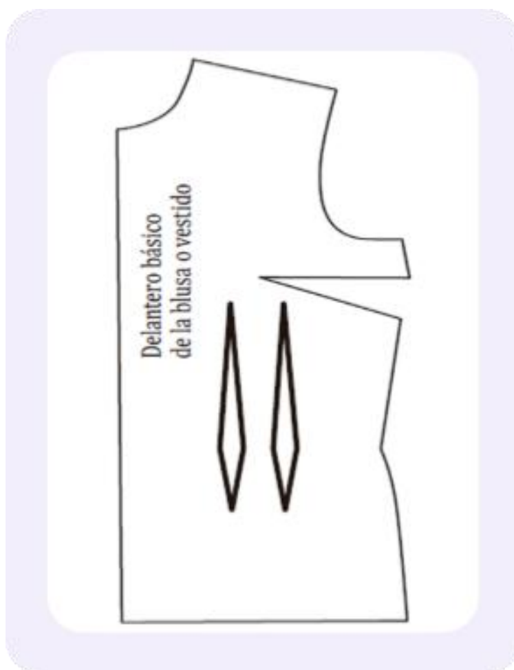
Figura 32. Sexto paso para el trazo
