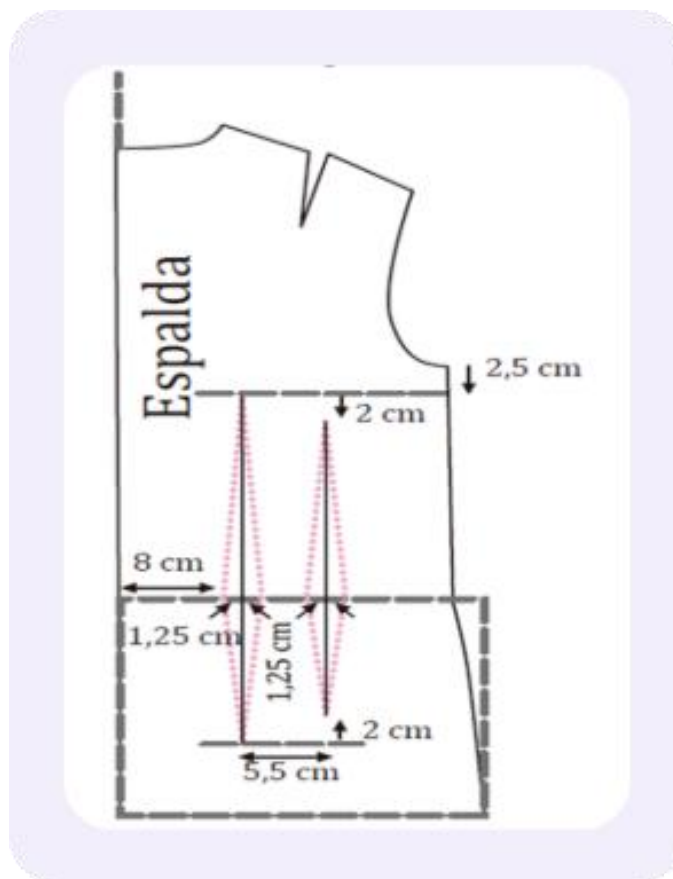
Figura 36. Décimo paso para el trazo
