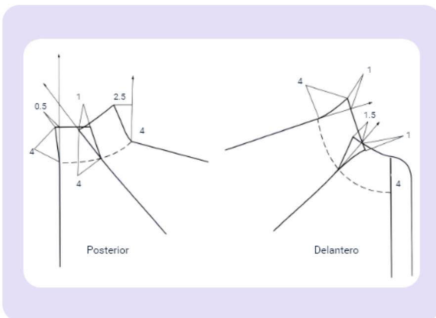
Figura 21. Cuello manga ranglán
