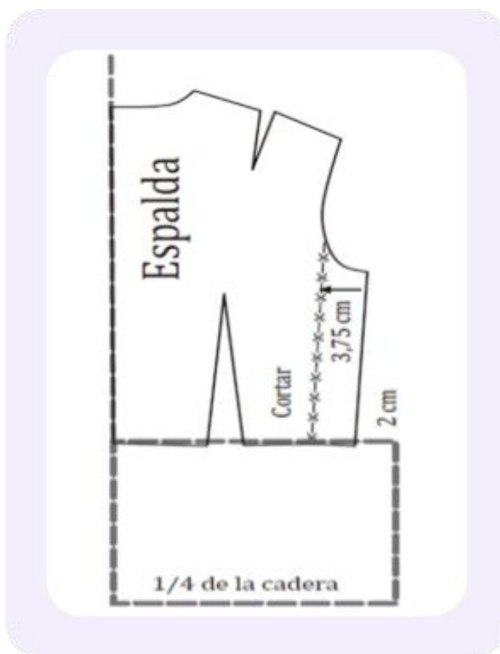
Figura 33. Séptimo paso para el trazo
