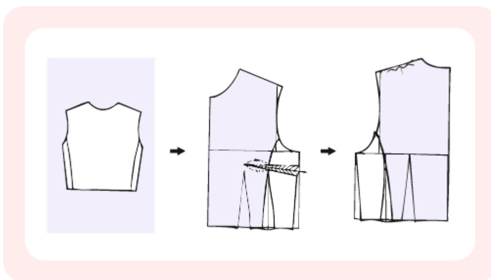
Figura 40. Crop top corte princesa en sisa corto
