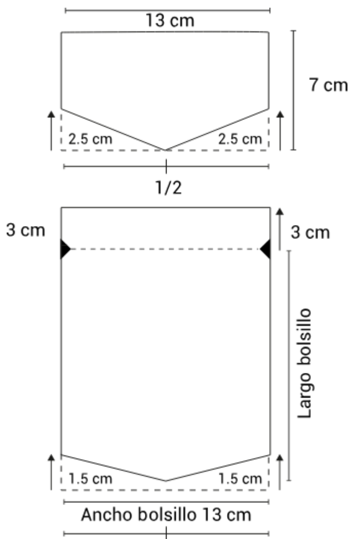
Figura 13. Trazo de bolsillo con tapa separada
