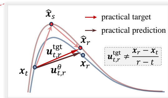
(d) practical learning of DTSC
