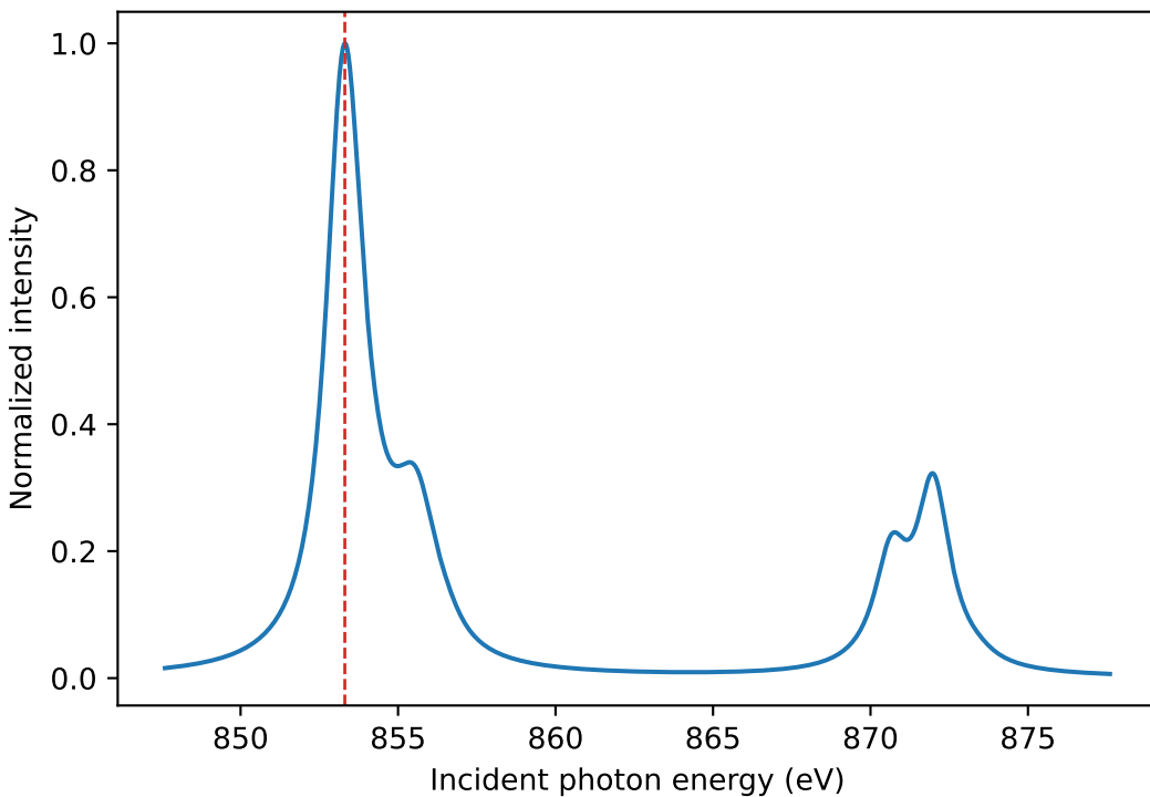
NiO L_{2,3} XAS
