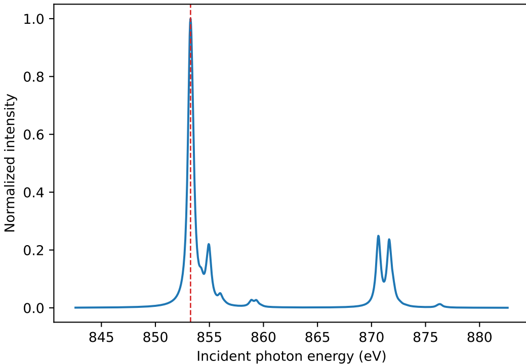
NiO SIAM XAS
