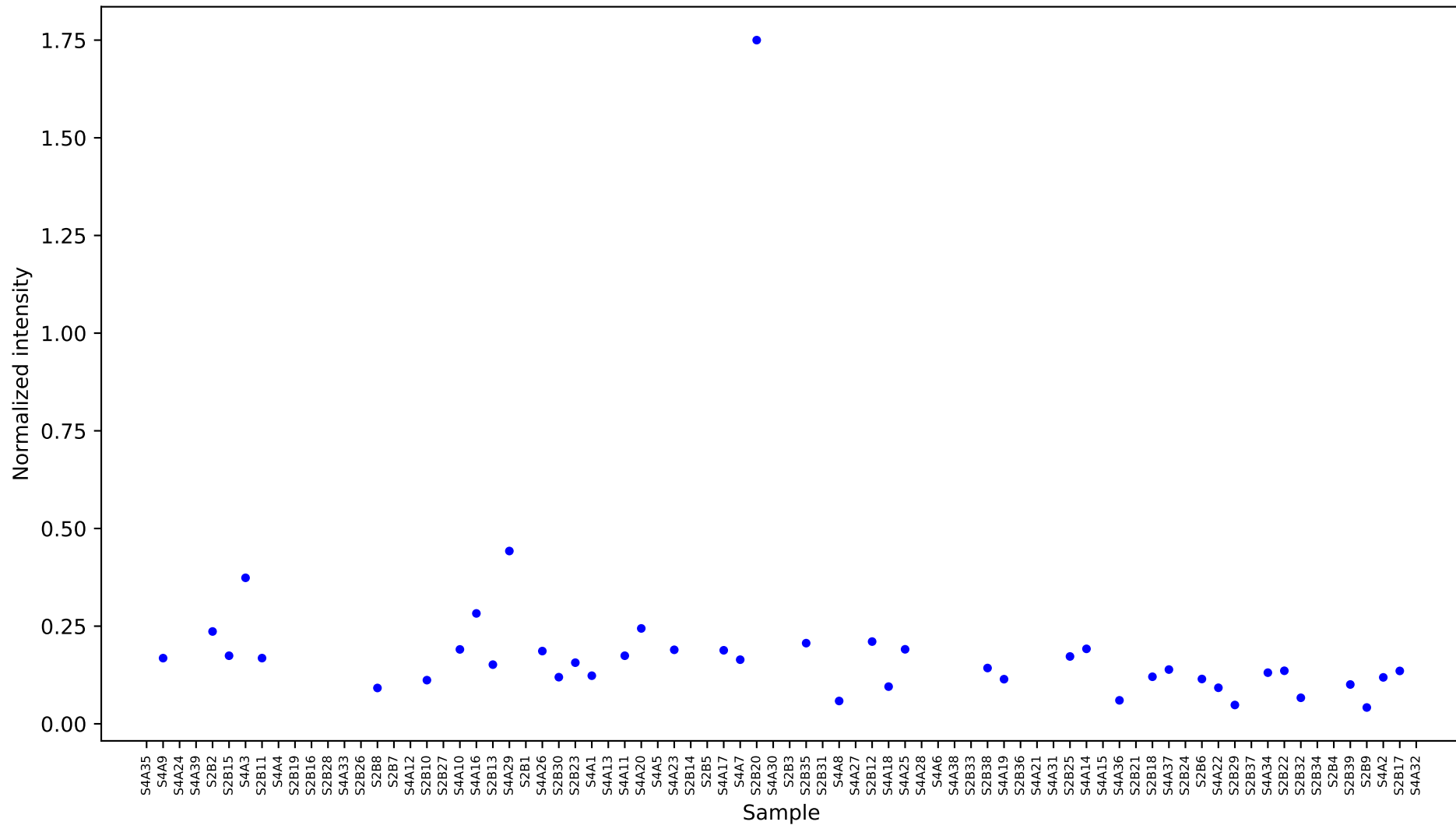
[236] L-asparagine 1 [14.496] Results.1
