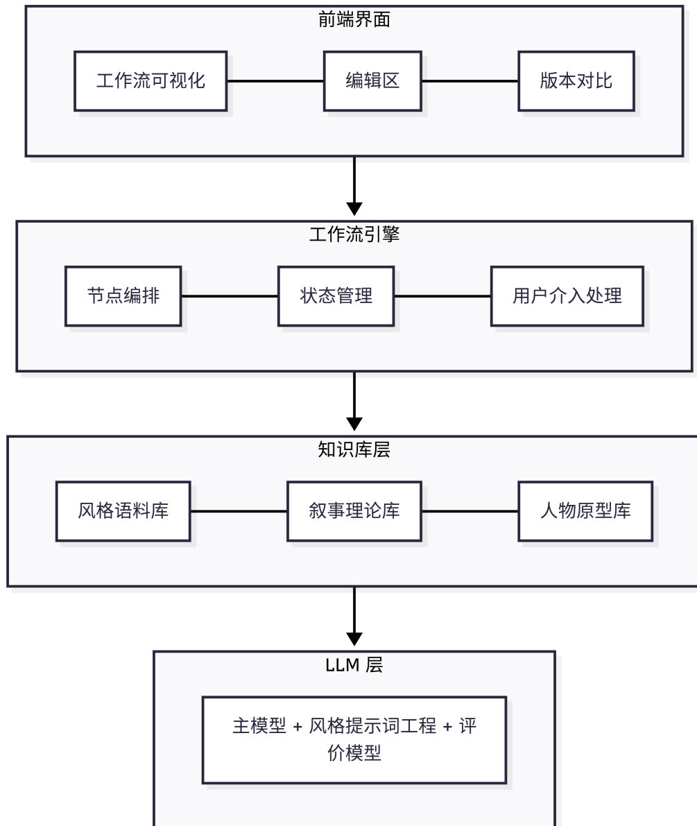
图 1: 文思工坊整体架构
