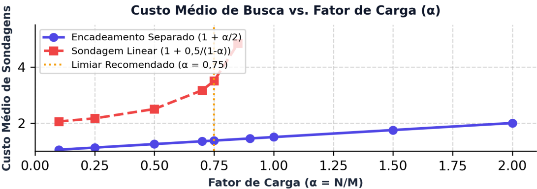
Figura 2: Curva teórica de degradação do número de sondagens/comparações em função do Fator de Carga (α).
