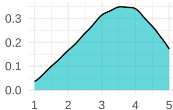
SOP
