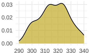
GRE.Score
