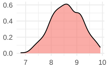
CGPA
