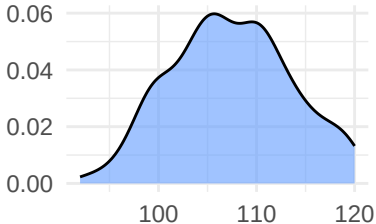
TOEFL.Score
