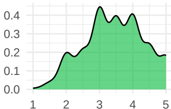
LOR
