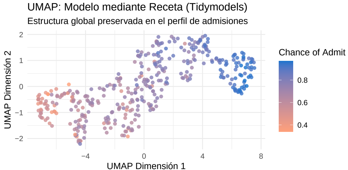
Figura 16: UMAP mediante receta tidymodels (step_umap)
