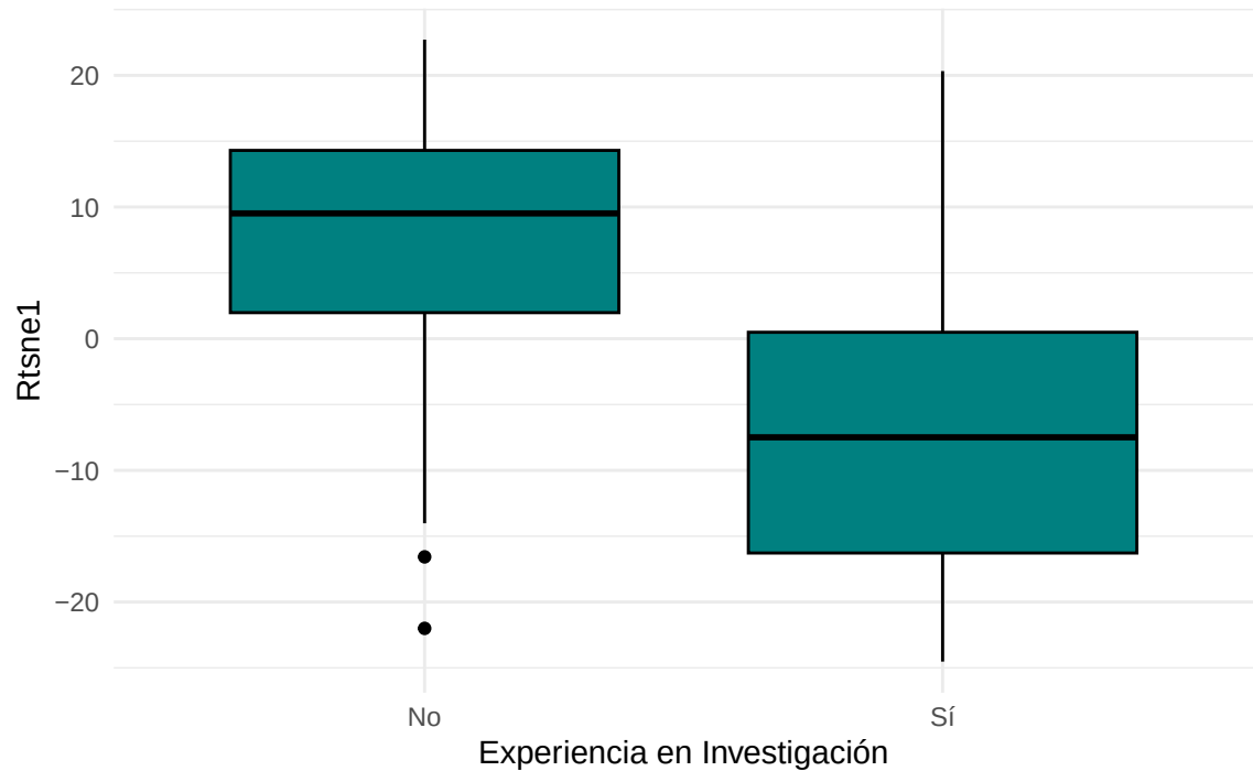
Distribución de Rtsne1 según Investigación
