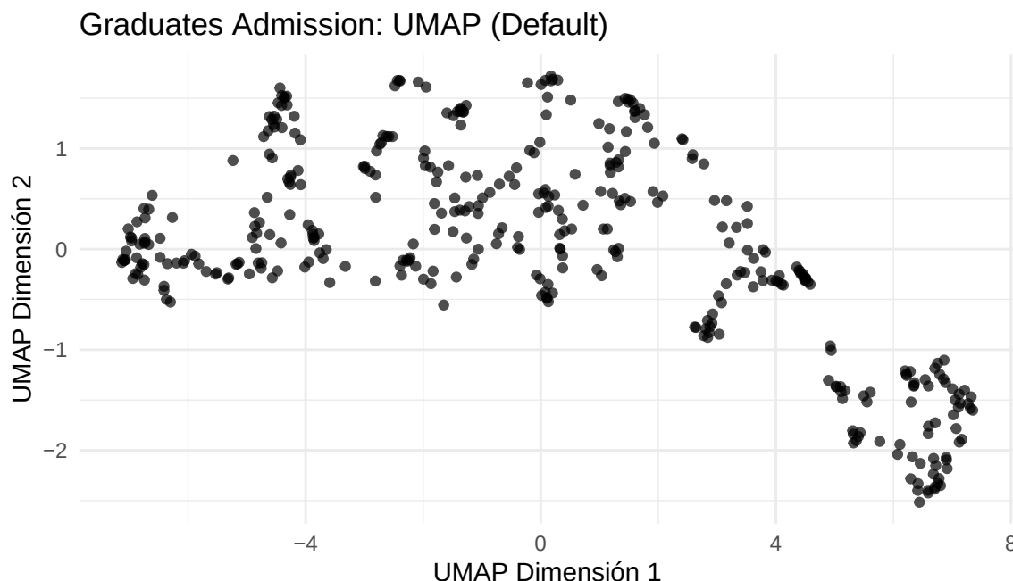
Figura 9: UMAP con configuración por defecto ( n_neighbors = 15 )
