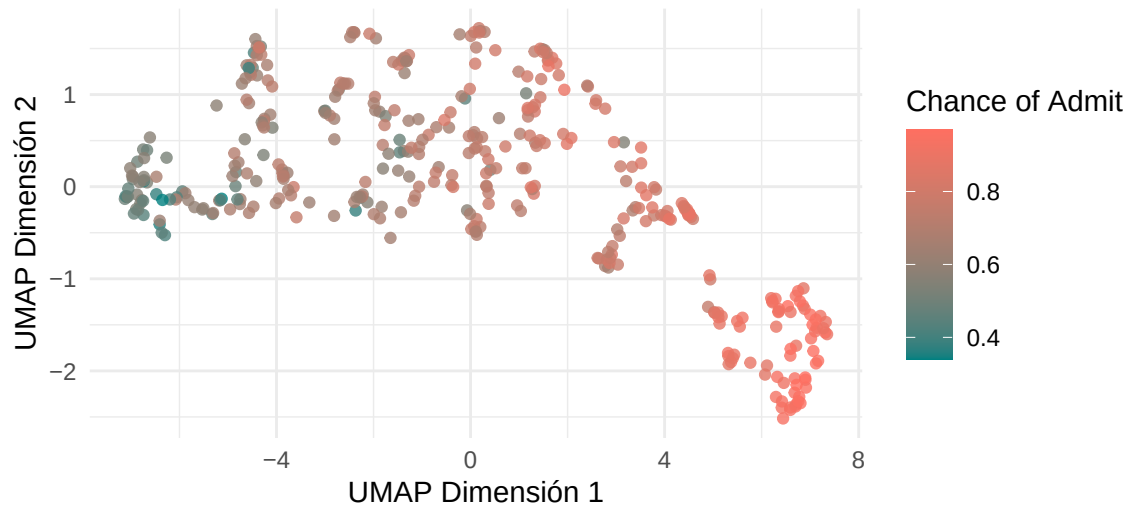
Figura 8: UMAP coloreado por la probabilidad de admisión, Chance of Admit
