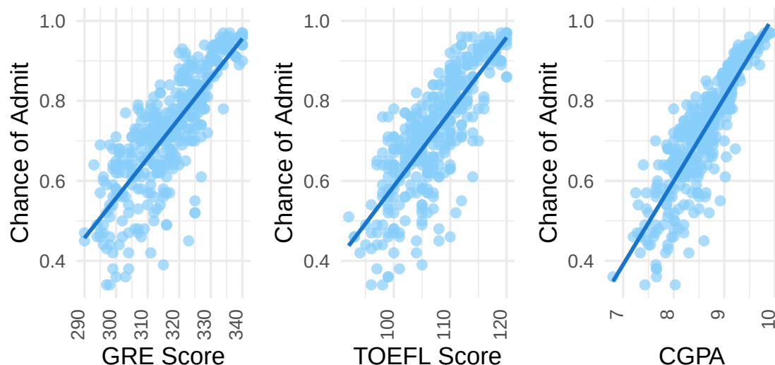
Figura 1: Relación entre las variables continuas y Chance of Admit
