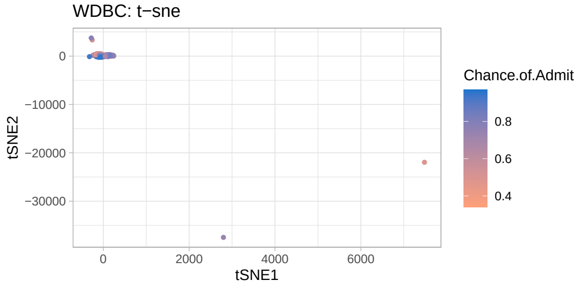
Figura 6: Salida de tsne() con parámetros por defecto, coloreada según Chance of Admit
