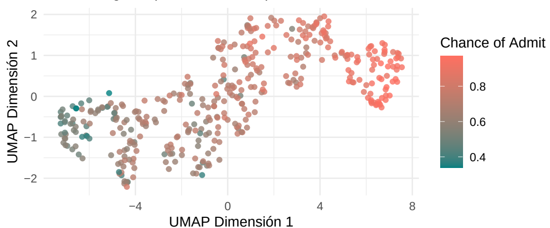
Figura 11: UMAP mediante receta tidymodels ( step_umap )
