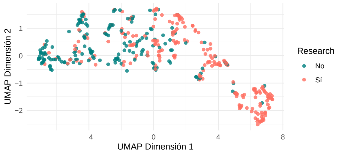
Figura 9: UMAP coloreado por experiencia en investigación, Research
