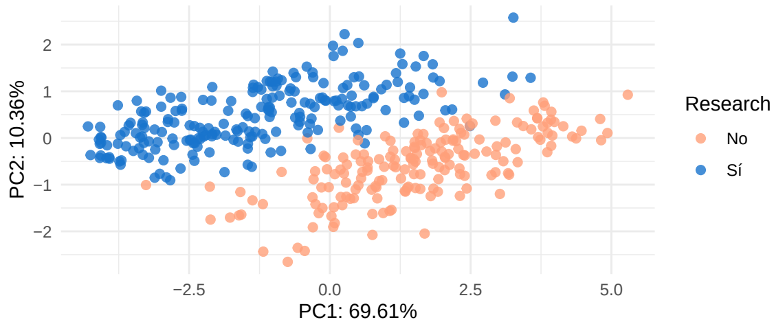
Figura 5: Proyección de los postulantes sobre PC1 y PC2, segmentada según experiencia en investigación
