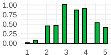
LOR
