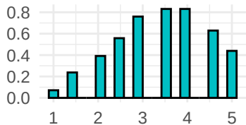
SOP
