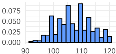
TOEFL.Score
