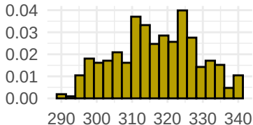
GRE.Score
