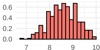
CGPA
