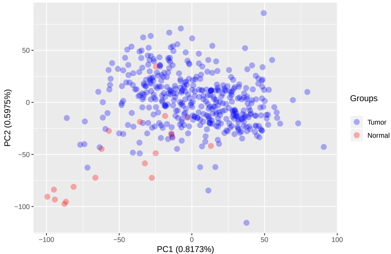
BLCA PCA
