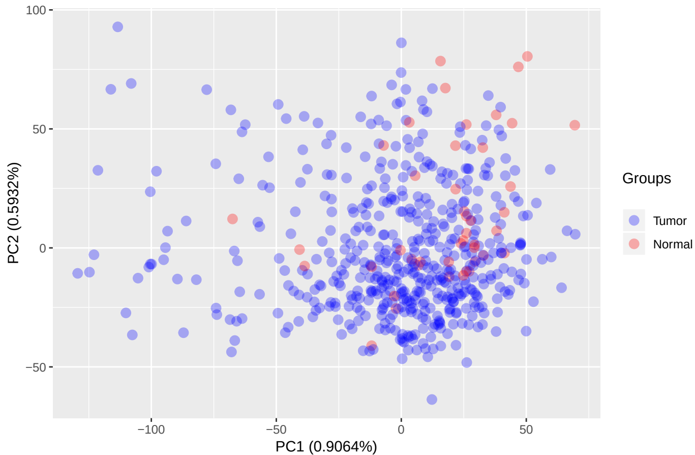
HNSC PCA
