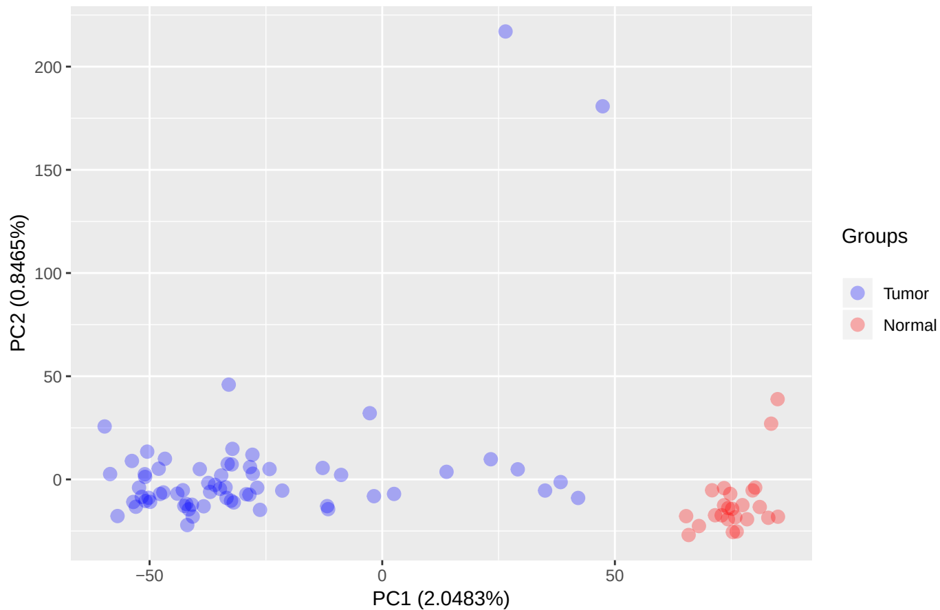
KICH PCA
