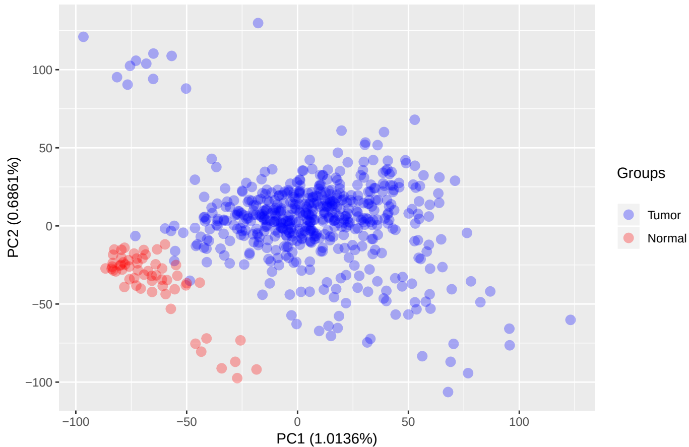
LUAD PCA
