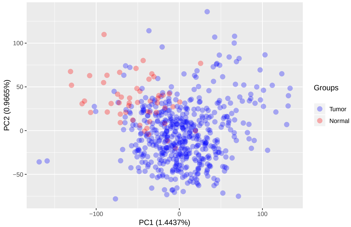
PRAD PCA
