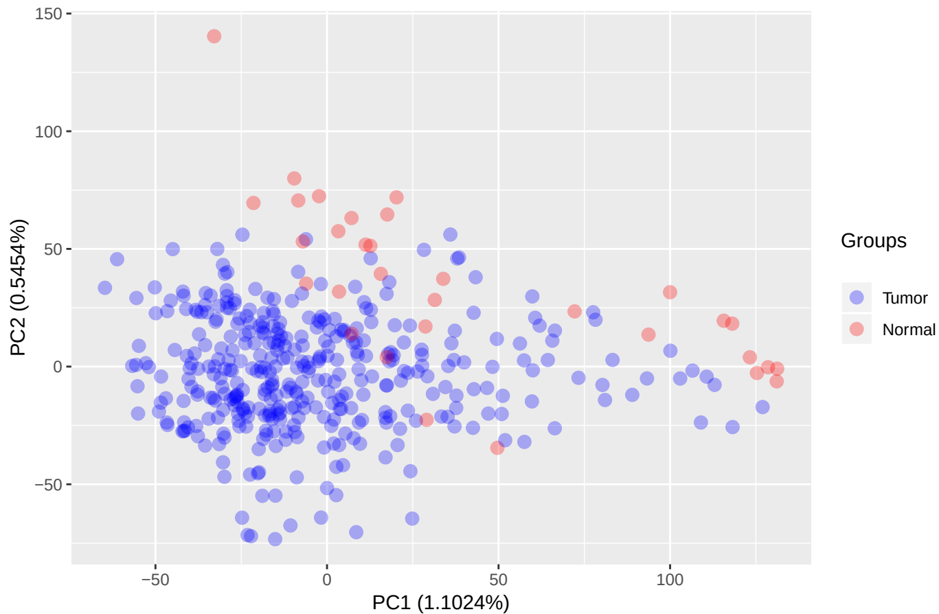
STAD PCA
