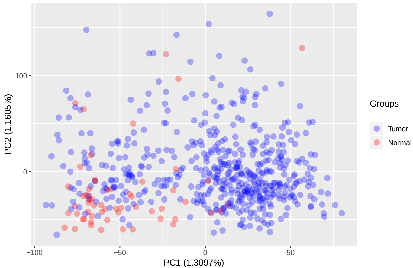
THCA PCA
