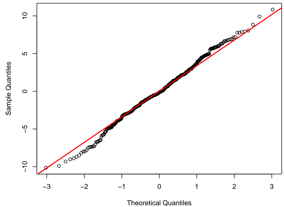
QQ-plot des résidus (Option 2)
