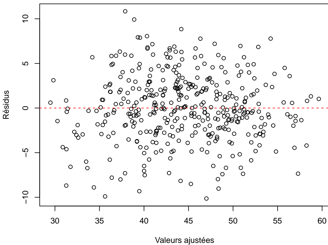
Résidus vs valeurs ajustées (Option 2)
