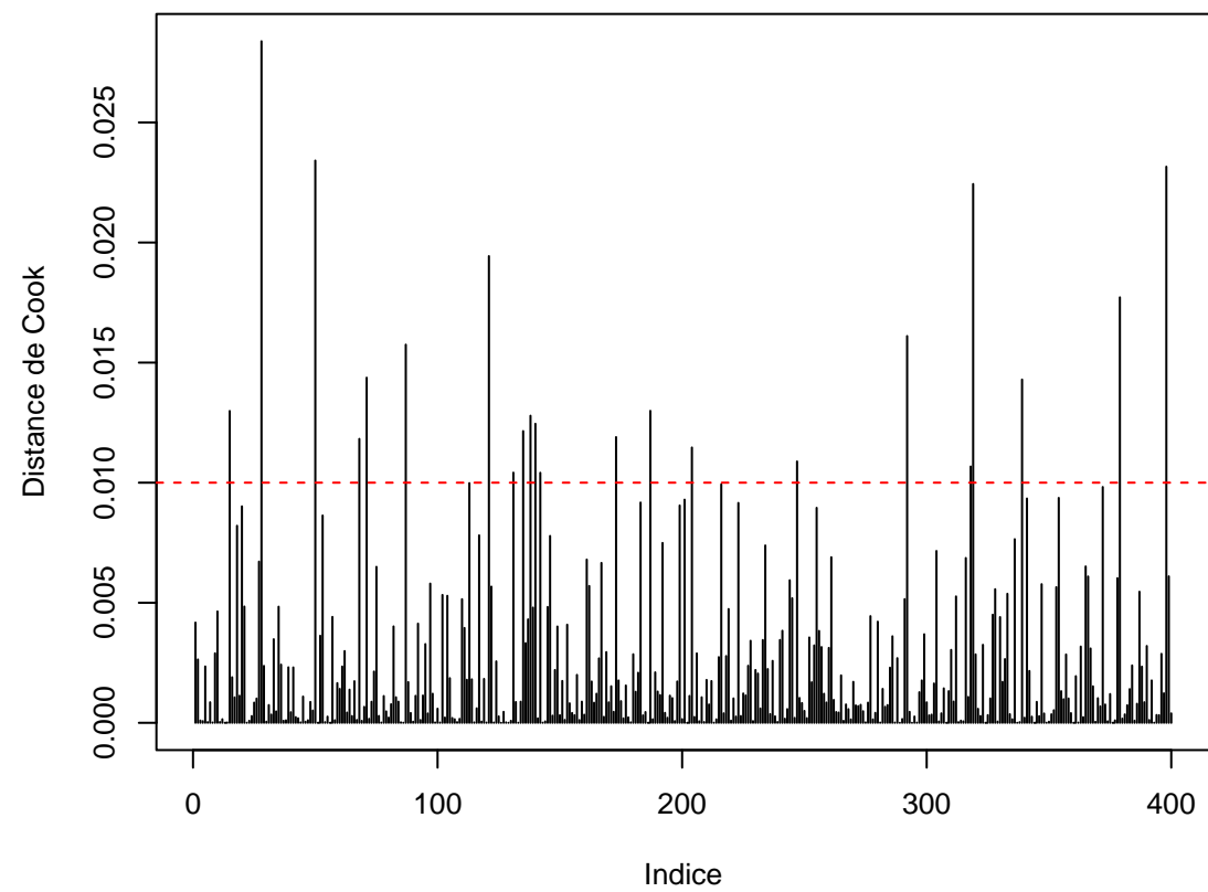
Distance de Cook
