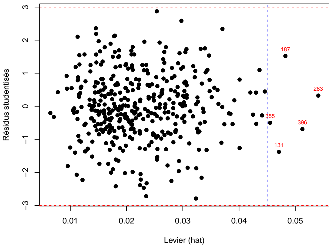
Levier vs Résidus studentisés
