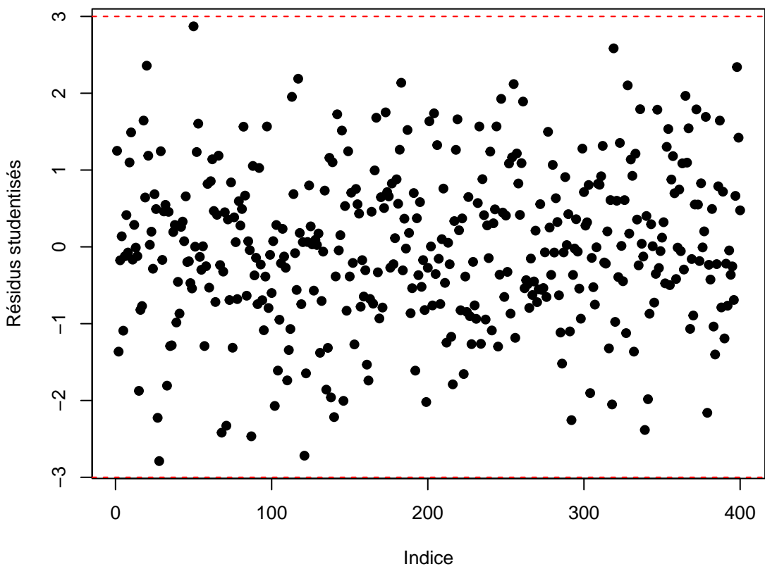
Résidus studentisés
