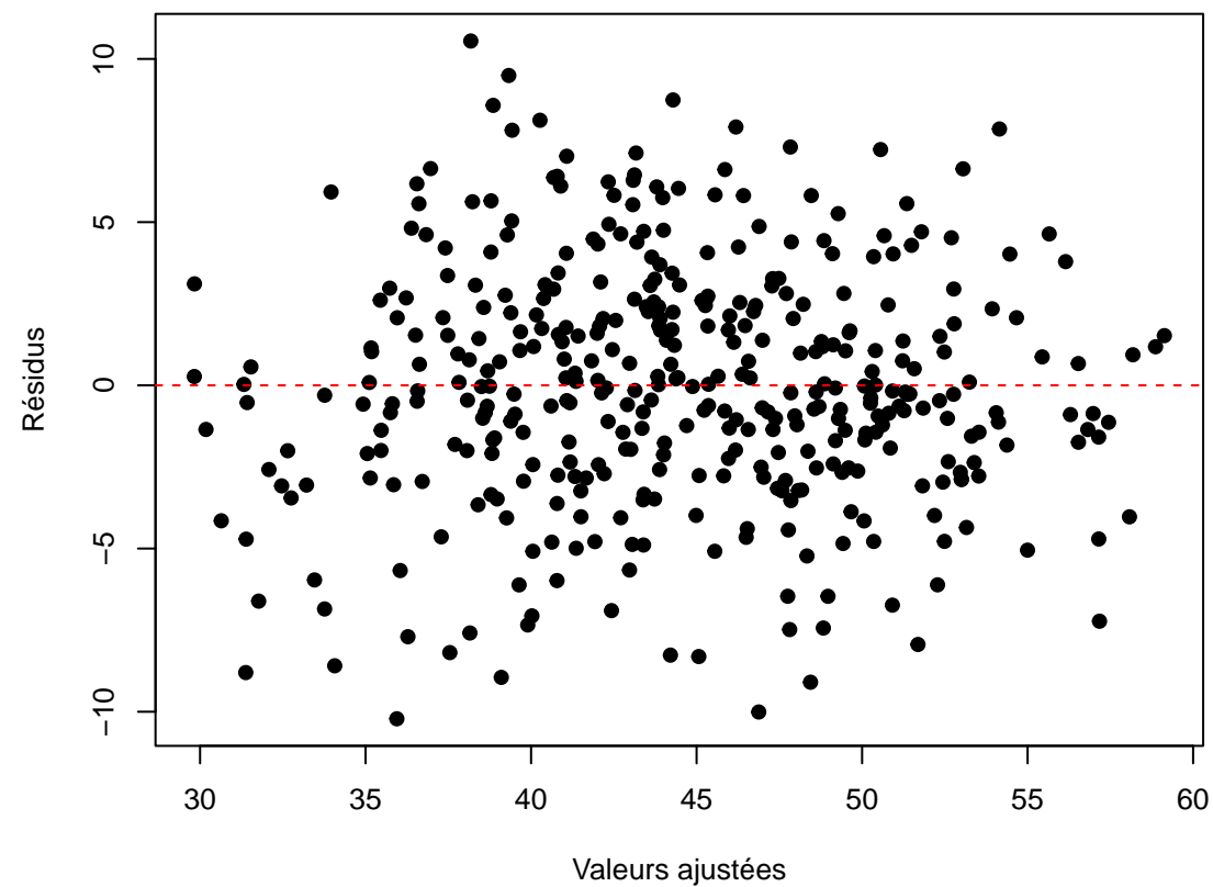
Résidus vs Valeurs ajustées
