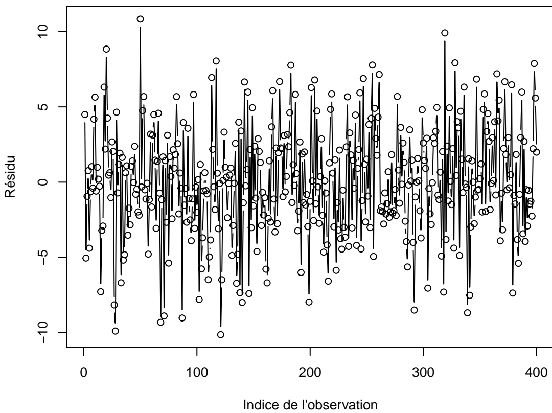
Résidus vs indice (Option 2)
