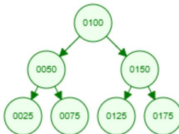
ABB de almacenes después del proceso de eliminación
