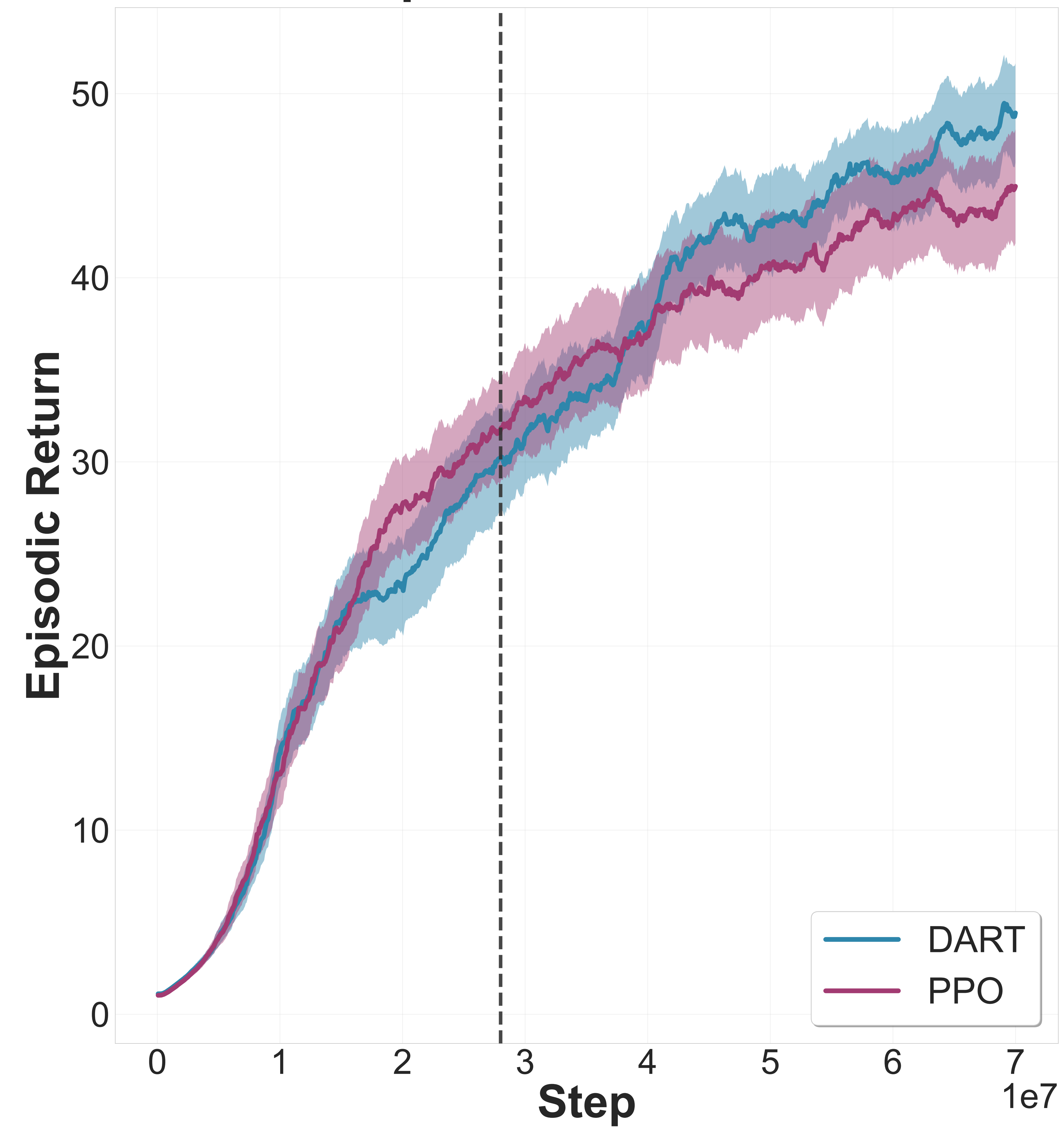
Sparse Humanoid
