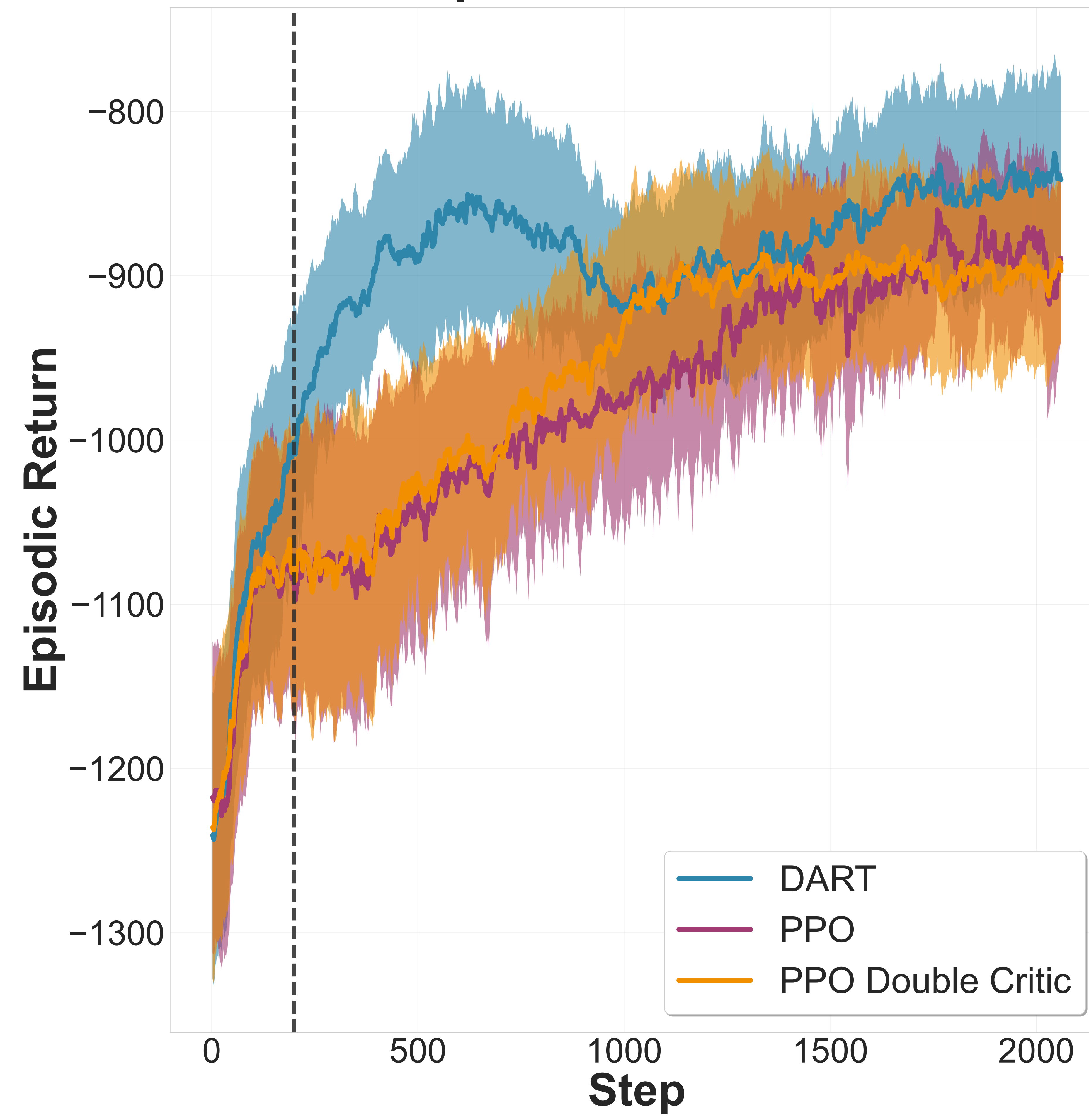
Sparse Pendulum
