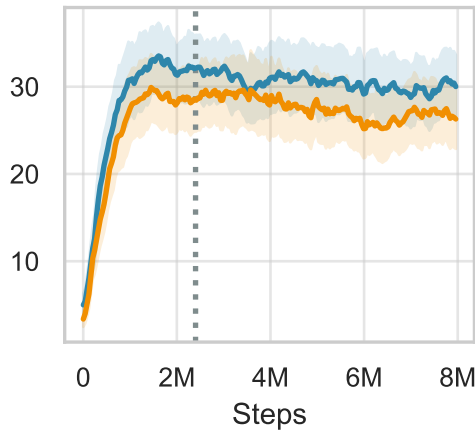
acrobot-swingup
