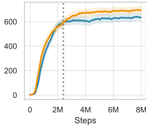
pendulum-swingup
