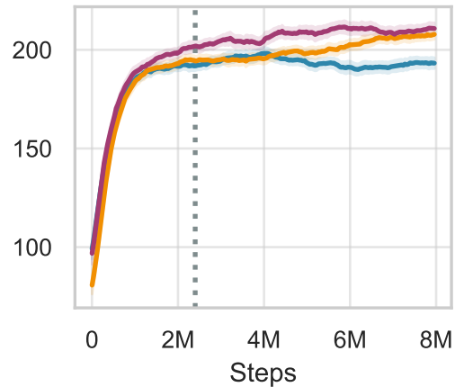
cartpole-two_poles
