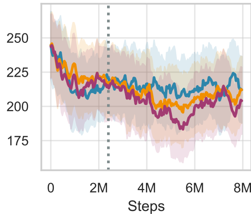
quadruped-fetch
