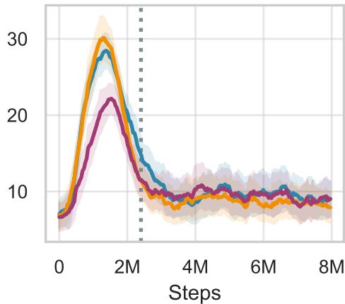
quadruped-escape
