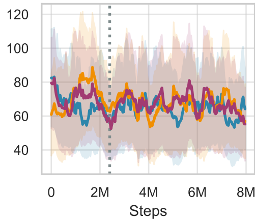
stacker-stack_2
