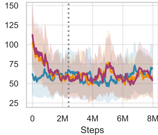
stacker-stack_4
