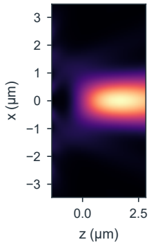
b TorchFDTD, |E|^2
