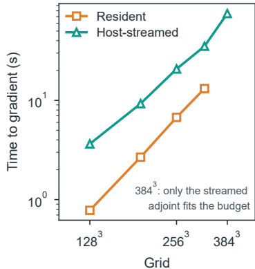
c Adjoint, 128 steps
