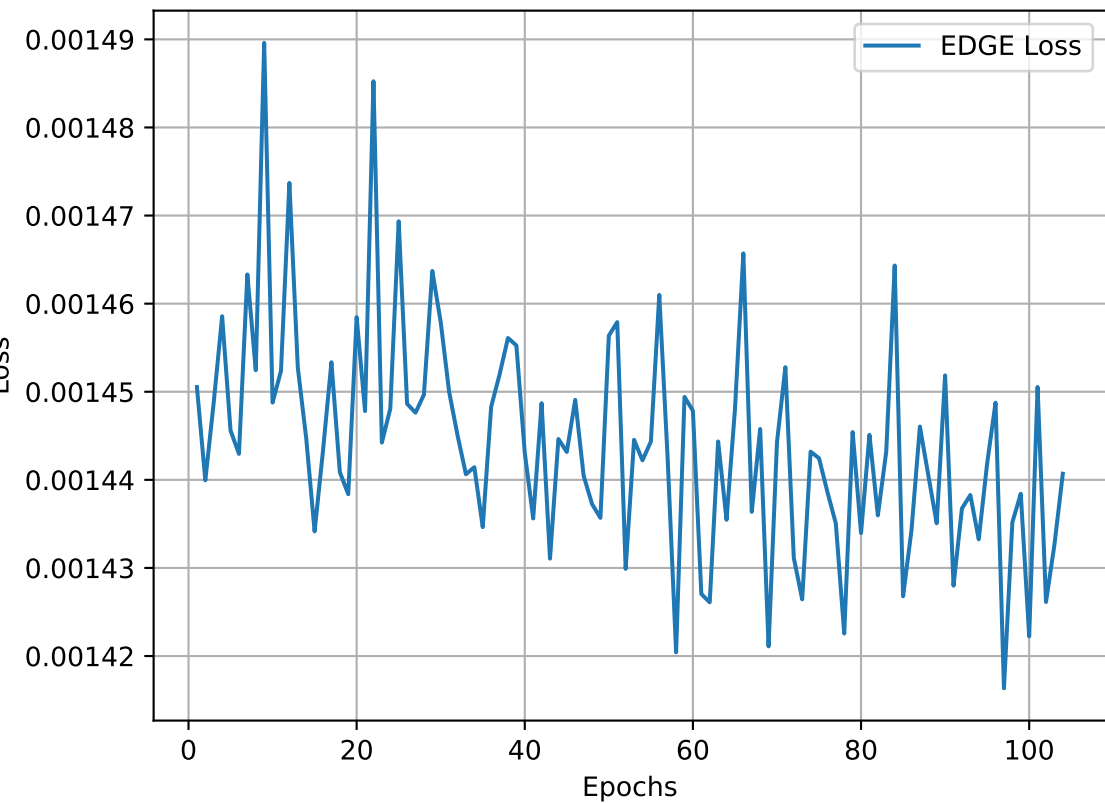
EDGE Loss
