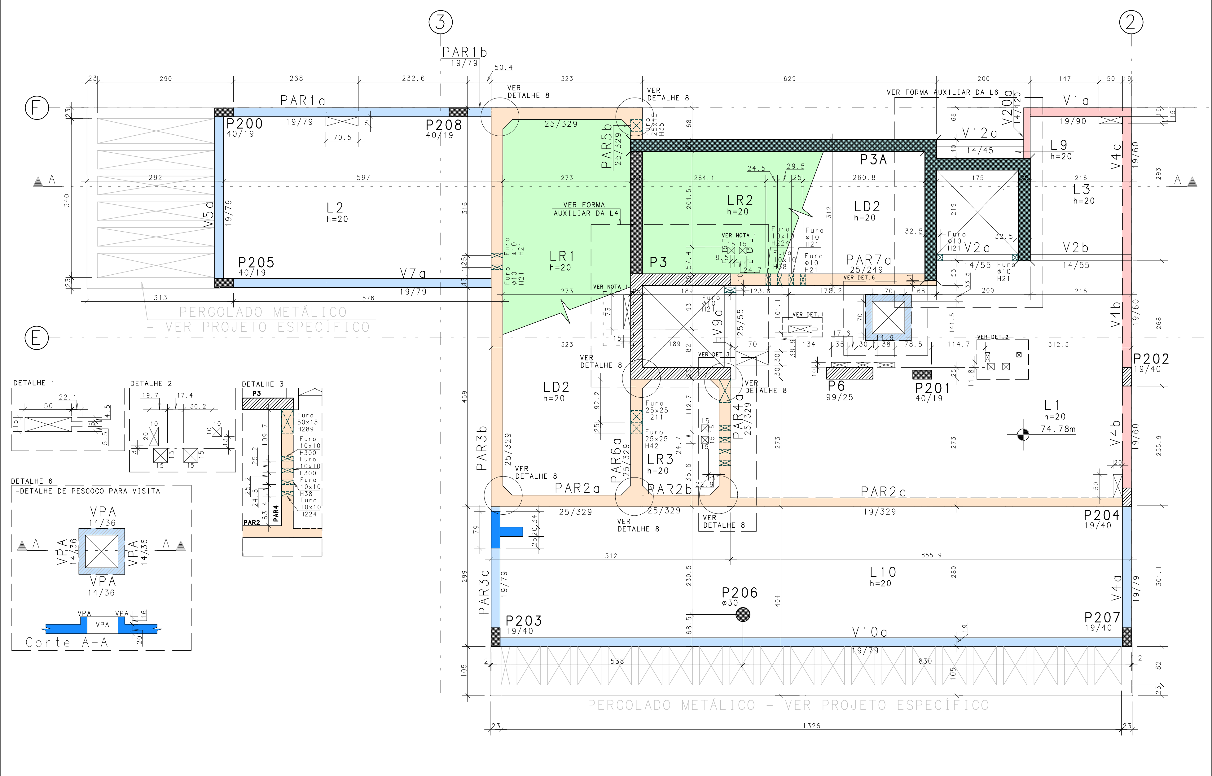
FORMA DO PAVIMENTO TÉCNICO (+74,78)
