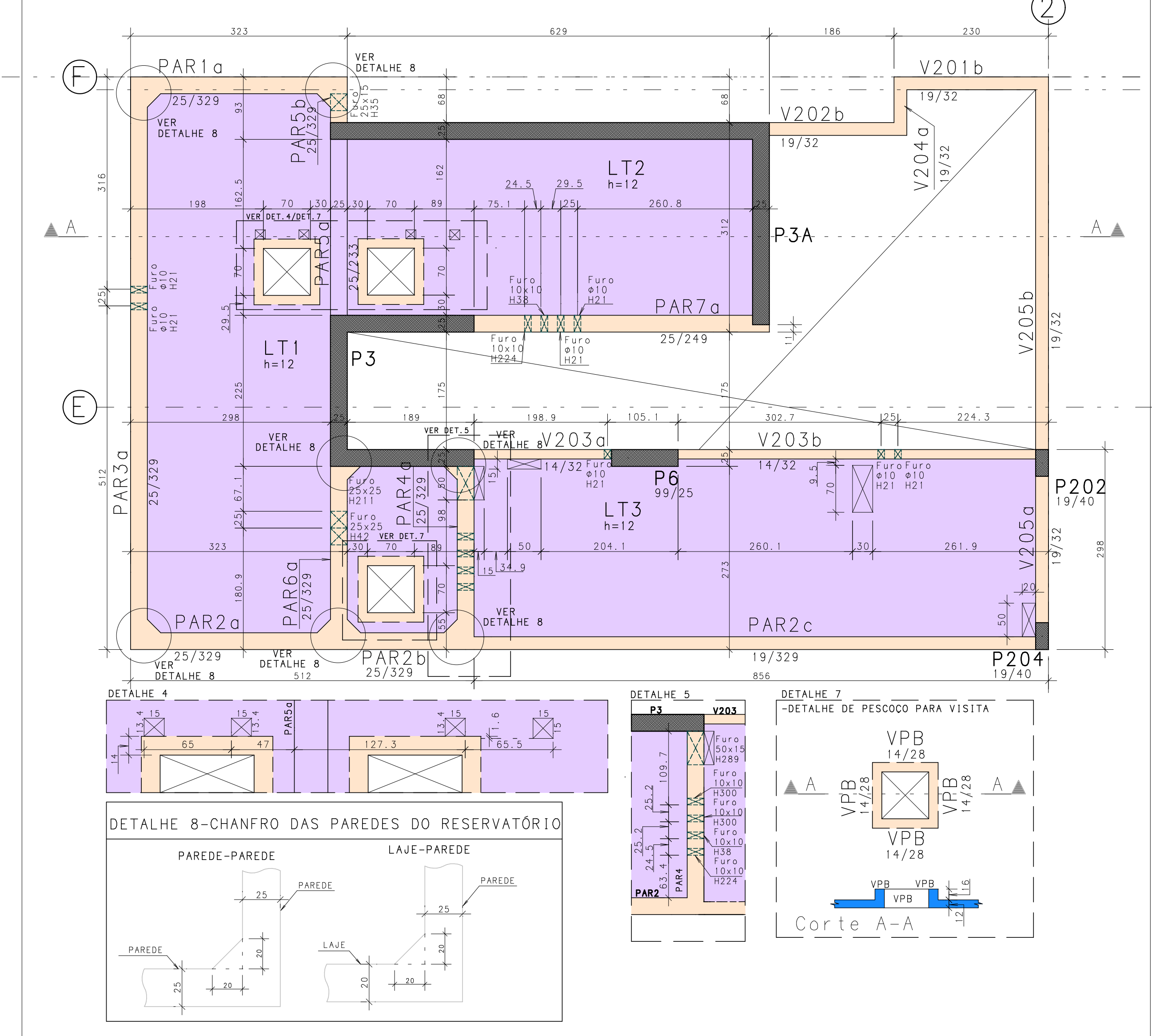
FORMA DO TELHADO (+77,71)
