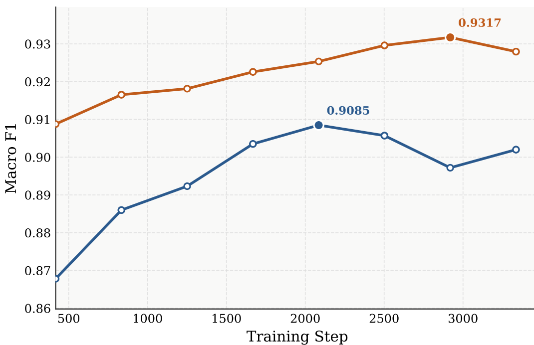
Validation Macro F1
