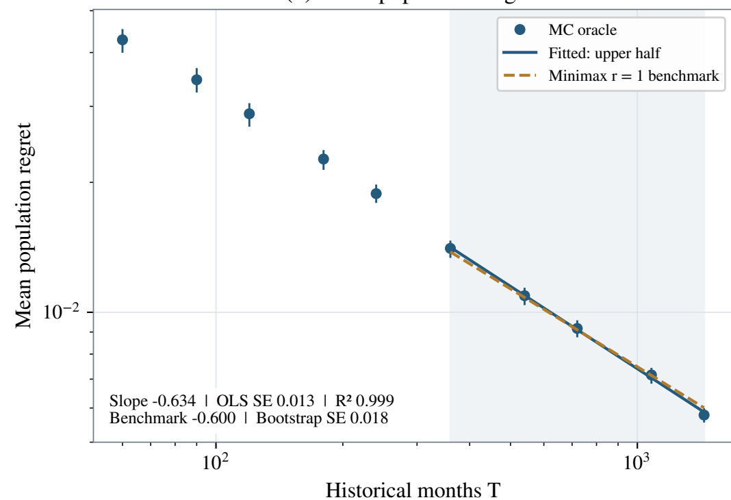
(d) Exact population regret
