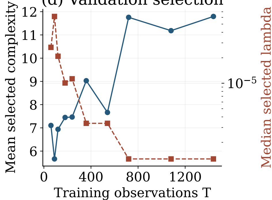
(d) Validation selection
