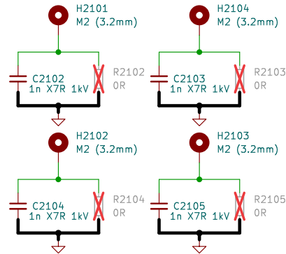
Module Holes
